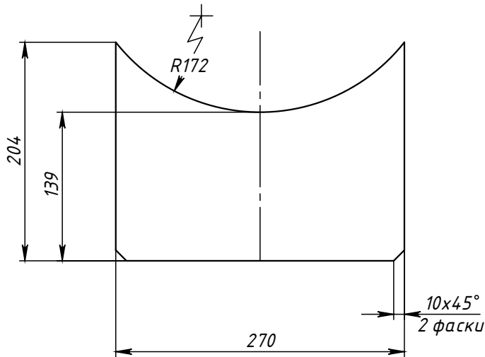
Поз.3 (Ребро)
